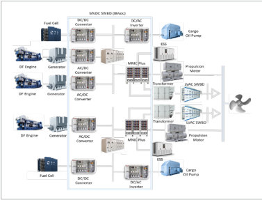
무탄소 전기추진 기본설계 개념도
